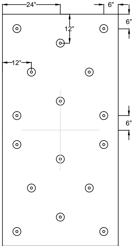
FIELD: 16 FASTNERS PER BOARD
